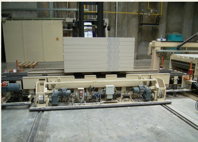
Querverfahrwagen mit Notaushub Cross Sliding Platform with Emergency Excavation
