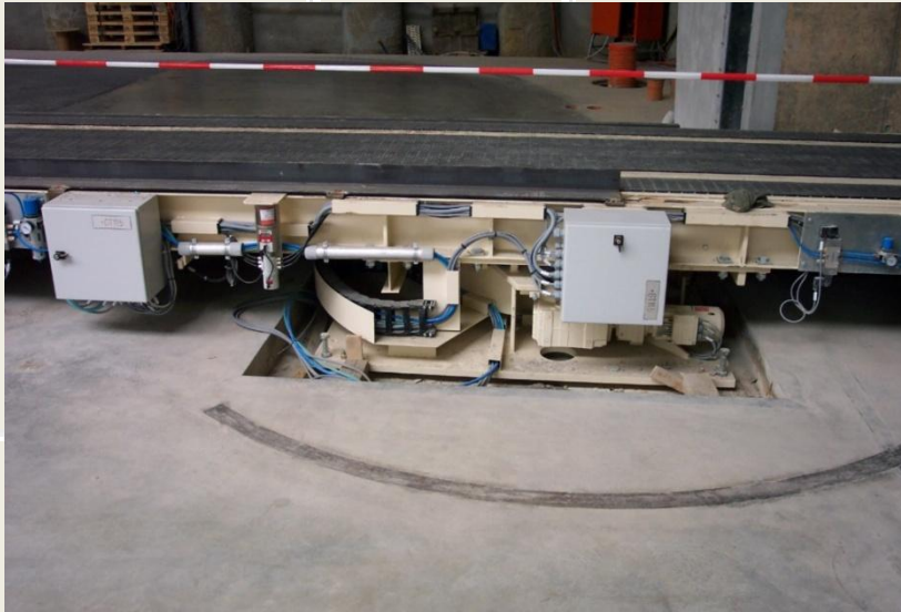
Modulbandförderer auf Drehteller Modular Belt Conveyor on Turntable
