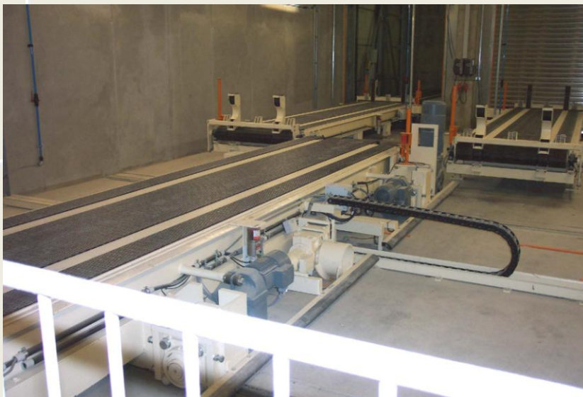
Querverfahrwagen zur Splittung in 2 Produktionslinien Cross Sliding Platform for Splitting to 2 Production Lines
