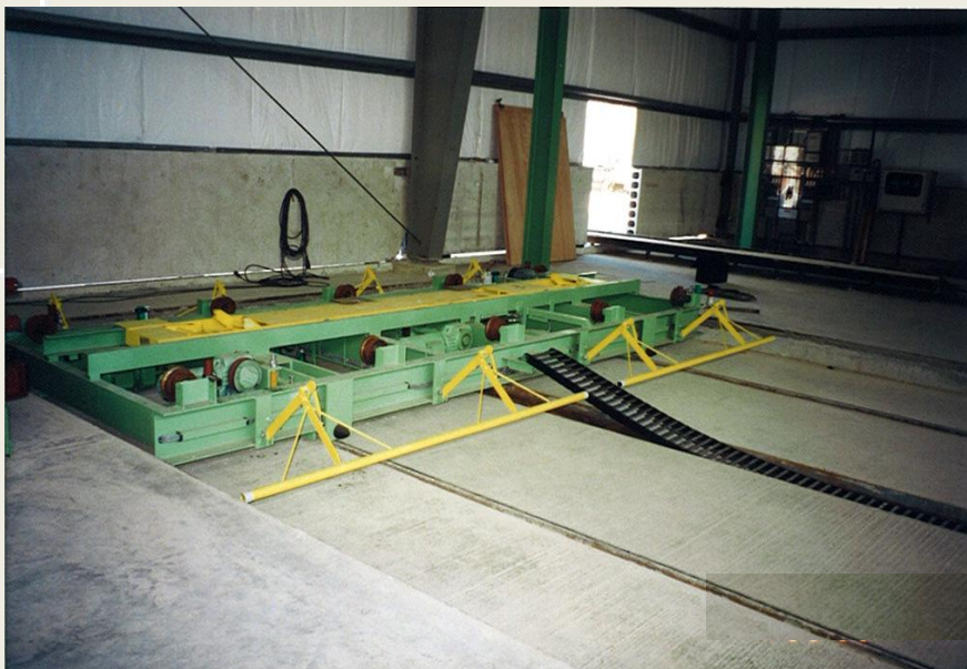
Schiebebühne mit Schubwagen und Reibrad Transfer Car with Push Car and Friction Gear
